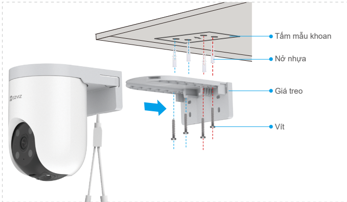
Hình 1 Gắn trần
